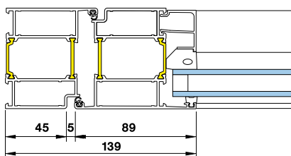
Стандартное дверное полотно
