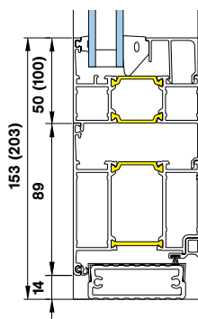
Неизолированный с RST поверхностью порог в двери с фальцем
