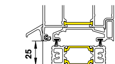
Изолированный порог в двери с щеточной прокладкой
