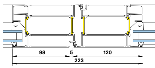
Двустворчатые двери с модульным профилем
