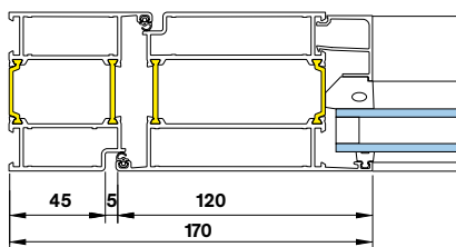
Модульное дверное полотно
