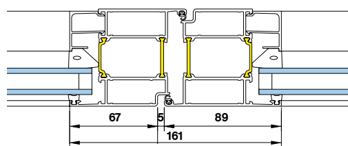
Двустворчатые двери со стандартным дверным профилем
