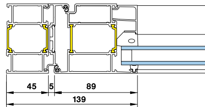
Стандартное дверное полотно со съемным фальцем
