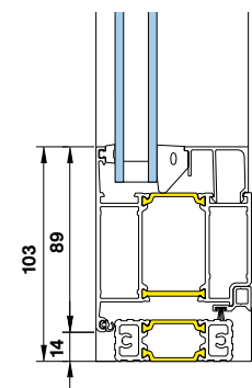
Изолированный порог в двери с фальцем
