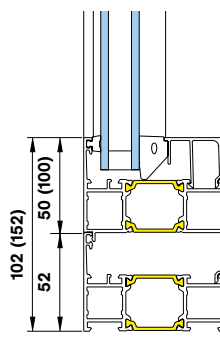
Боковая часть фиксированной двери с высоким профилем
