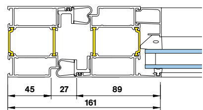
Стандартный или модульный профиль для двери с защитой от удара по пальцам
