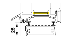
Неизолированный порог в двери с щеточной прокладкой
