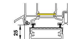
Неизолированный с RST поверхностью порог в двери с щеточной прокладкой
